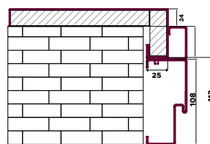
Portal z ościeżnicą regulowaną IRON
