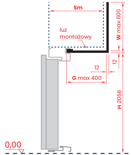
PRZEKRÓJ PIONOWY
