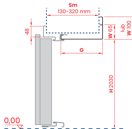
PRZEKRÓJ PIONOWY
