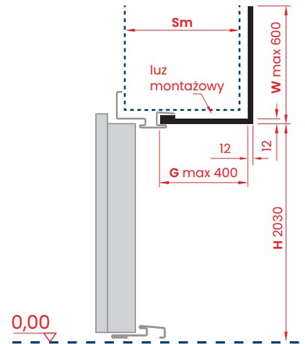
PRZEKRÓJ PIONOWY
