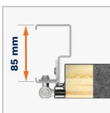
Ościeżnica stalowa FB
