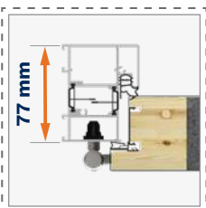
Ościeżnica ALUTHERM 60*
