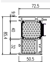
Rysunek techniczny
