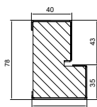
Rysunek techniczny
