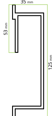
przekrój
